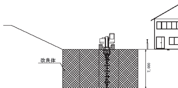
図 4.1-3 施工断面
