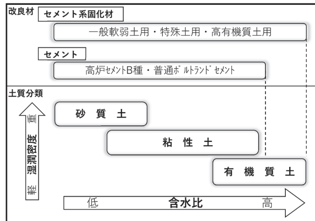
図 2.3-3 土質に対する改良材選定概念図
