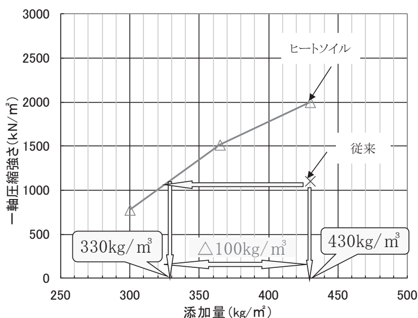
図 2.3-5 ヒートソイルの室内配合試験結果による添加量削減の可能性
