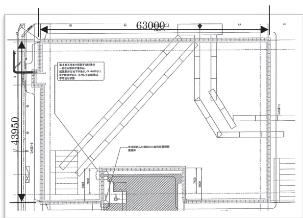
図 1.4-1 現場平面図
