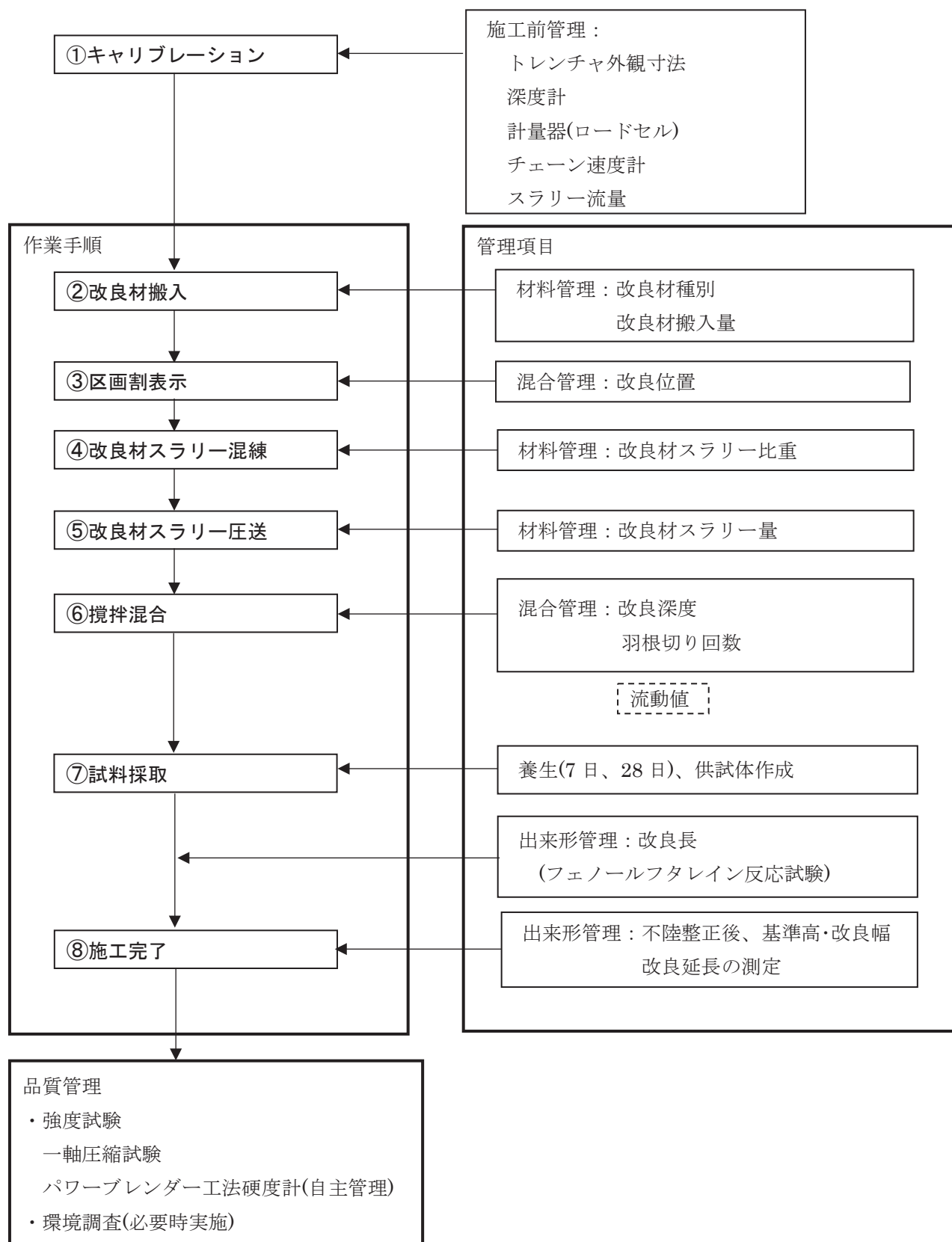
図 3.4-1 施工手順及び管理項目
