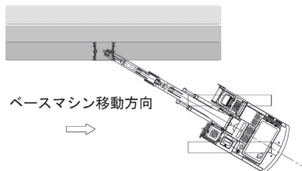
図 1.1-2 施工平面図
