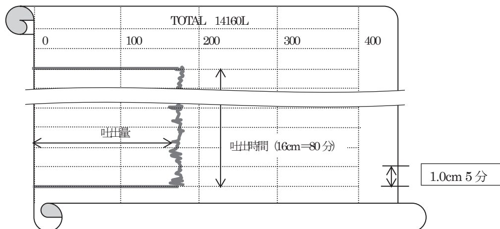
図 3.4-2 スラリーチャート紙模式図
