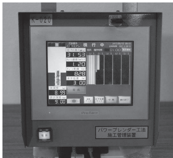
写真 3.4-1 施工管理装置
