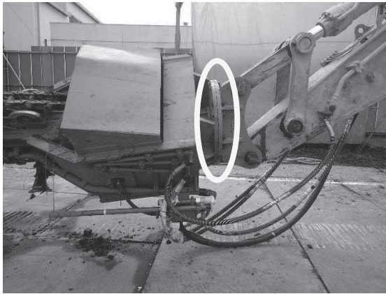
写真 1.2-1 角度変換機能部
