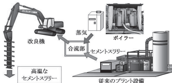
図 2.1-1 ヒートソイル工法のセメントスラリー高温化システム
