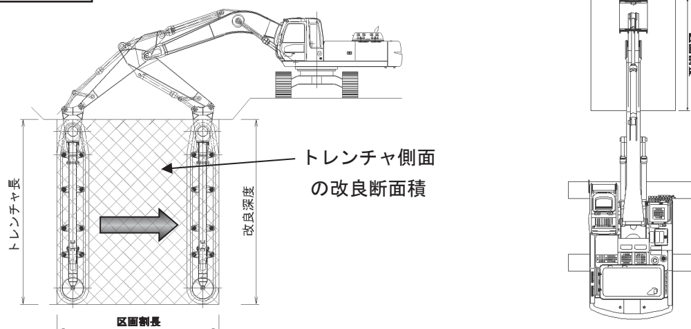
図 3.4-6 トレンチャ攪拌翼の羽根切り回数に用いる諸元
