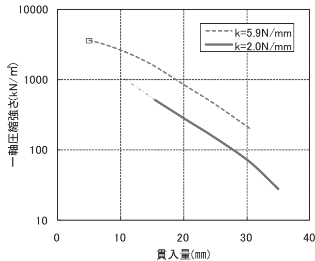
図 3.4-10 硬度計貫入量と一軸圧縮強さの相関
