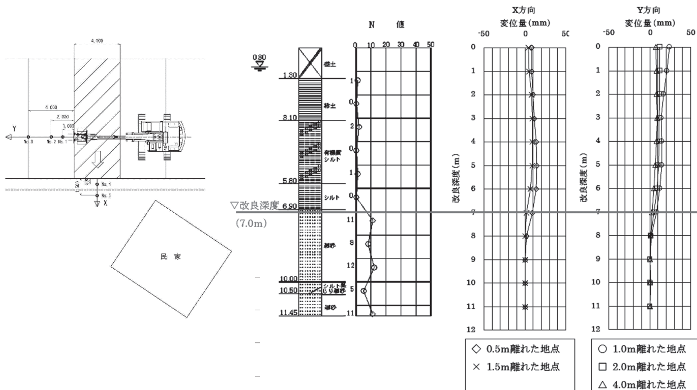
図 4.1-4 改良に伴う地中変位の計測例 (現場 No. 7)
