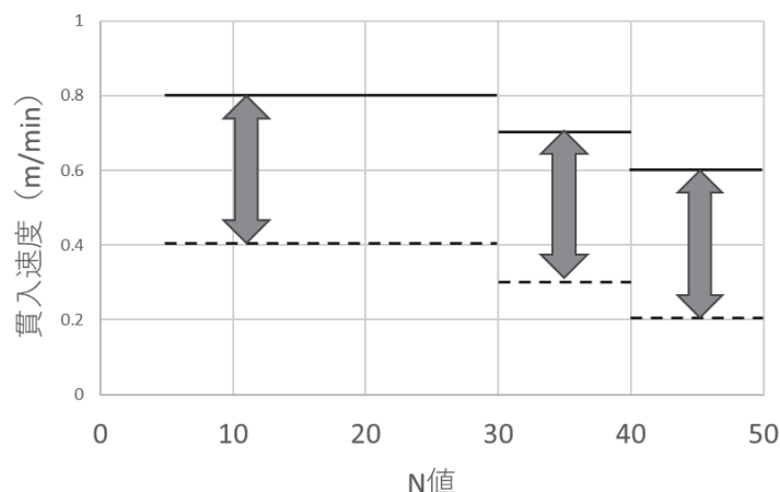
図 3. 6-2 目標着底層の N 値とトレンチャ貫入速度の目安
