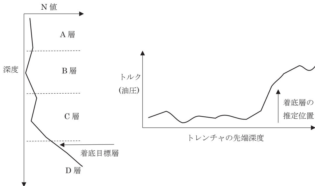
図 3.6-1 トレンチを一定速度で貫入させたときのトルク変化のイメージ
