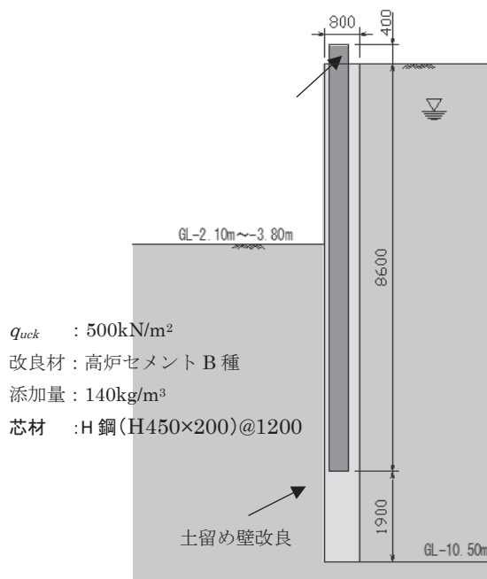
図 1.4-2 土留緒元
