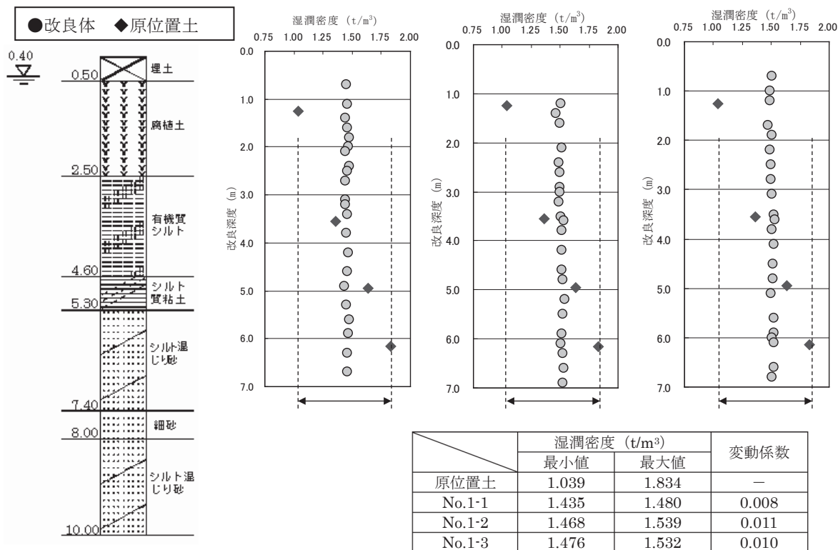
図 3.7-1 未改良土と改良土の湿潤密度の比較
