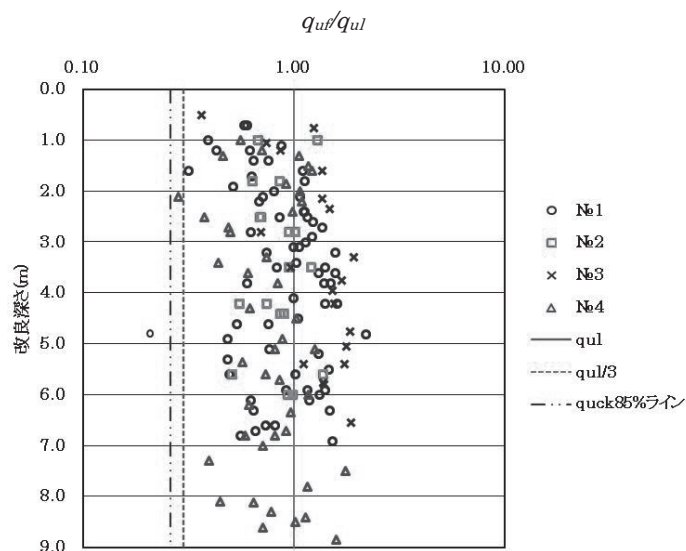
図 3.7-3 深度方向における現場強度( q_{uf} )と室内強度の平均値( \overline{q_{ul}} )の比
