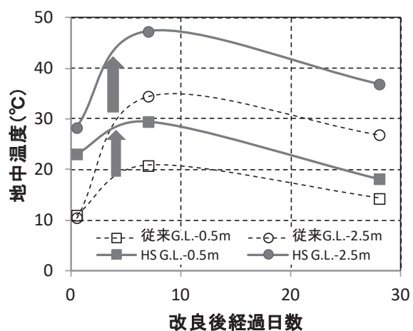
図 2.3-2 改良後経過日数と地中温度の関係
