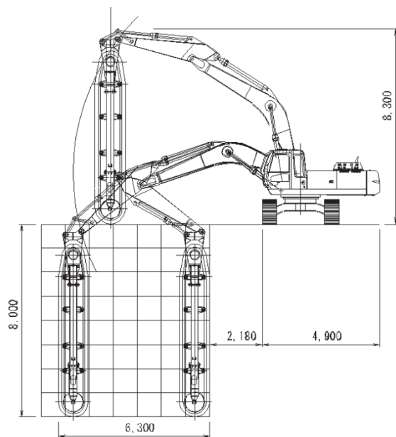
1.4m 3 クラス PBT-700
