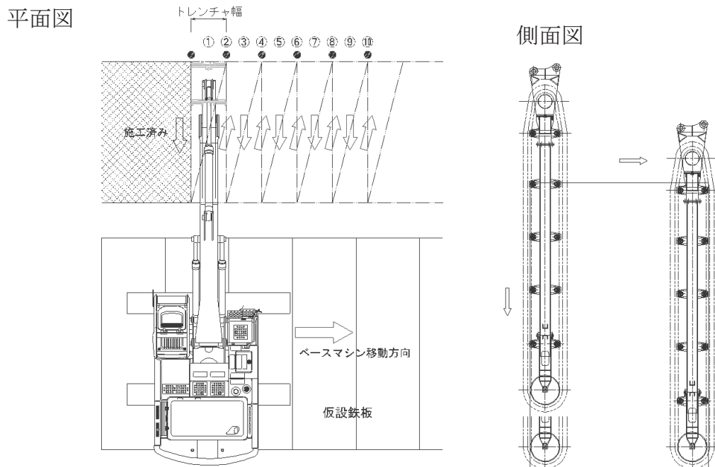
図 3. 3-1 N 字施工の手順図
