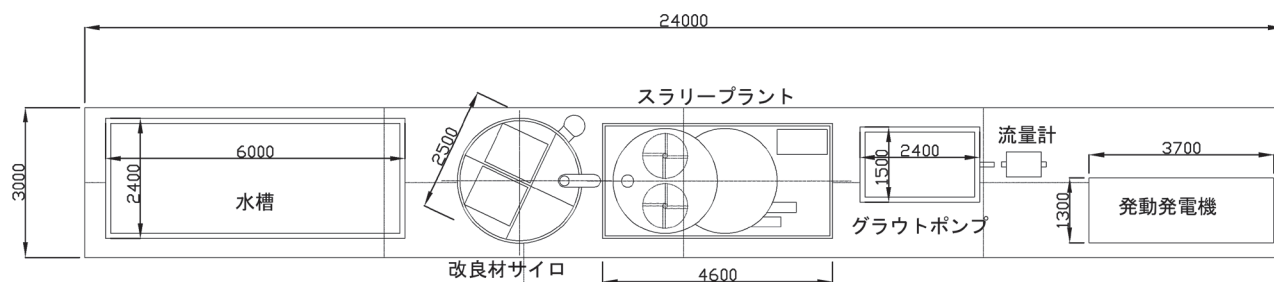
図 3.2-3 スラリープラントの設置例②（定置式プラント）
