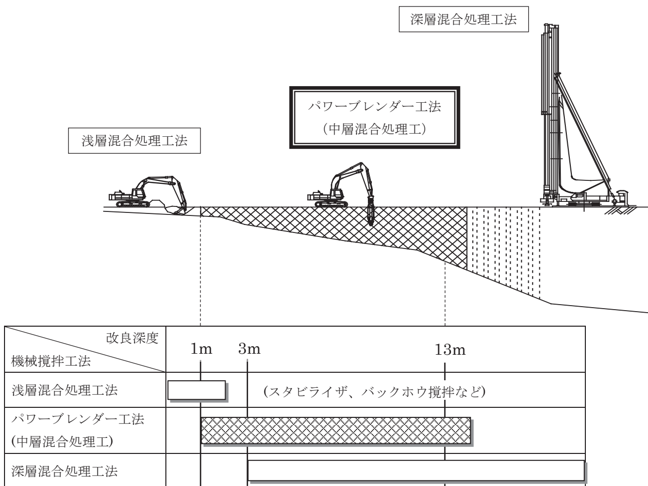
図 1.3-1 機械撹拌の固化系混合処理工法と改良深度
