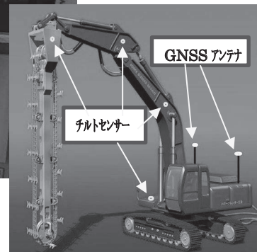
ICT 活用による地盤改良
