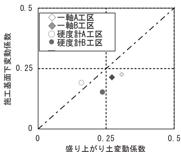
図 3.9-2 平均値変動係数の比較
