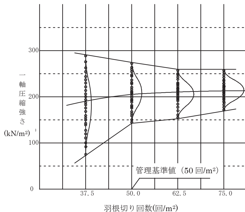
図 3.4-4 羽根切り回数と一軸圧縮強さの実験データ
