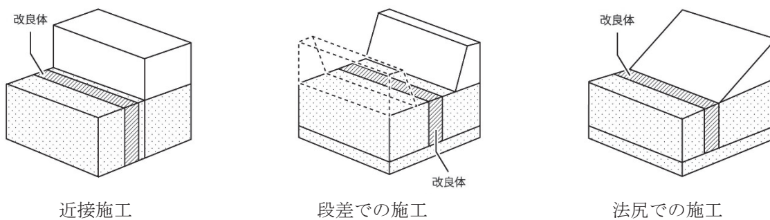
図 1.3-2 現場条件による適用例
