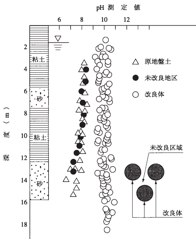
図 4.3-1 pH 測定 (例) 1)
