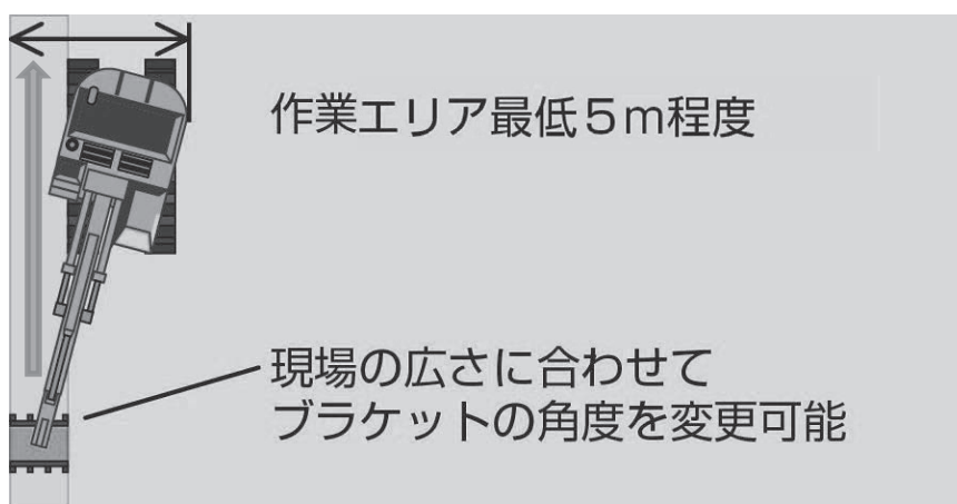
図 1.3-3 最小作業エリア図
