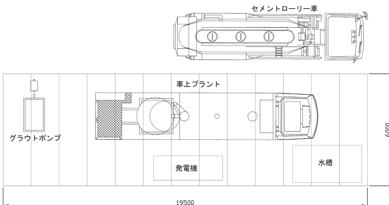
図 3.2-4 スラリープラントの設置例（車載式・セメントローリー車）
